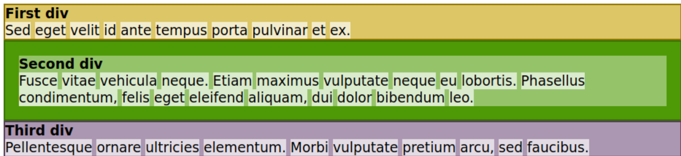
Figure 37. Des conteneurs div différents peuvent avoir des padding différents.
